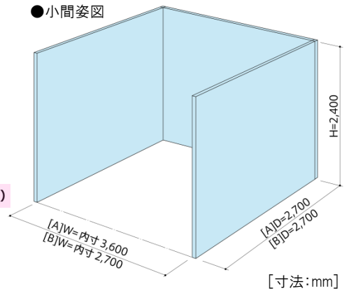
●小間姿図
